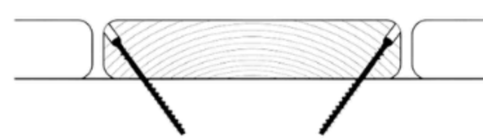
Installation 45 degrés
